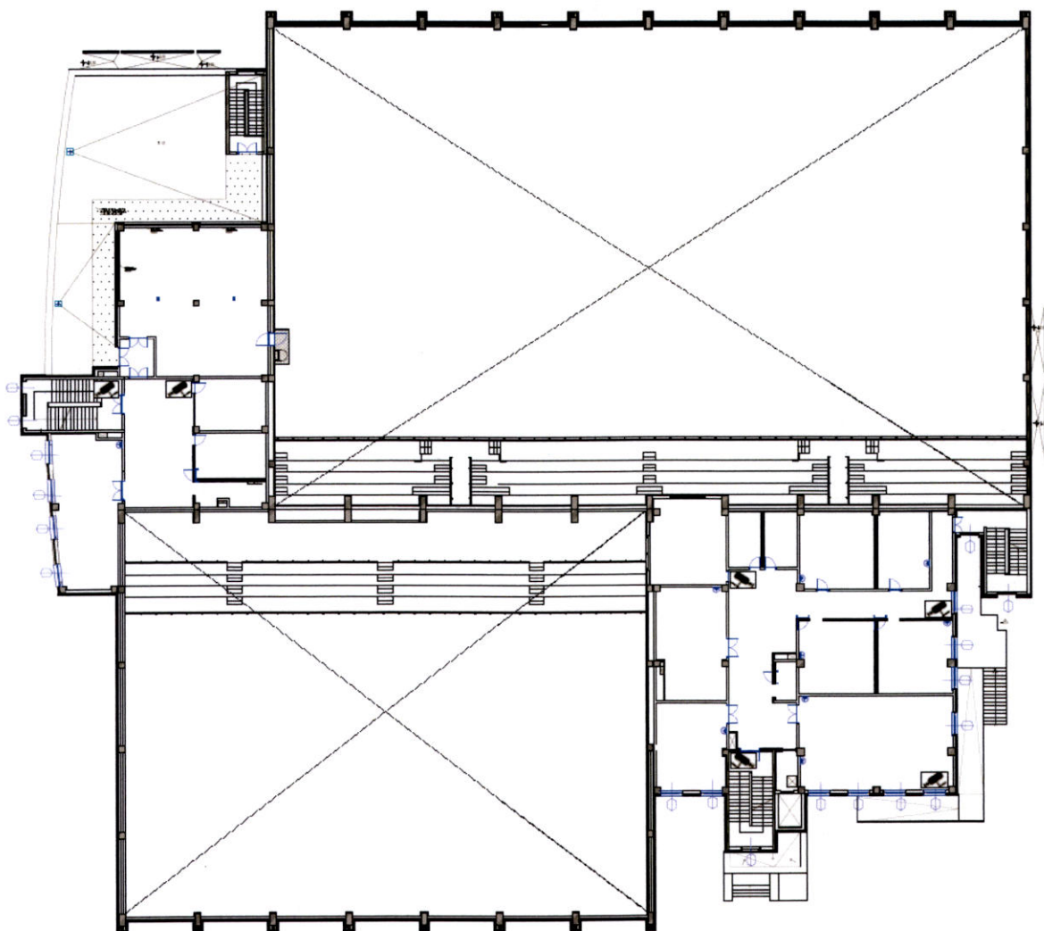
План четвертого этажа
